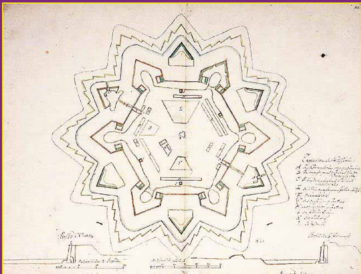
Plánek věznice Leopoldov z 19. století (foto: Wikipedie)
