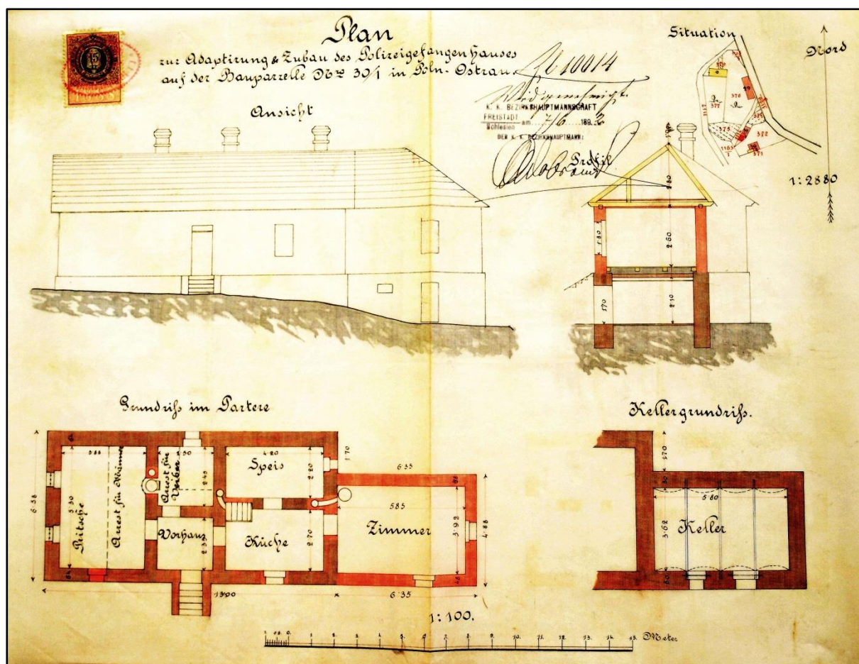
Plán na přestavbu věznice v Polské Ostravě z roku 1892 (foto: SOkA Karviná, f. Okresní úřad Fryštát)
