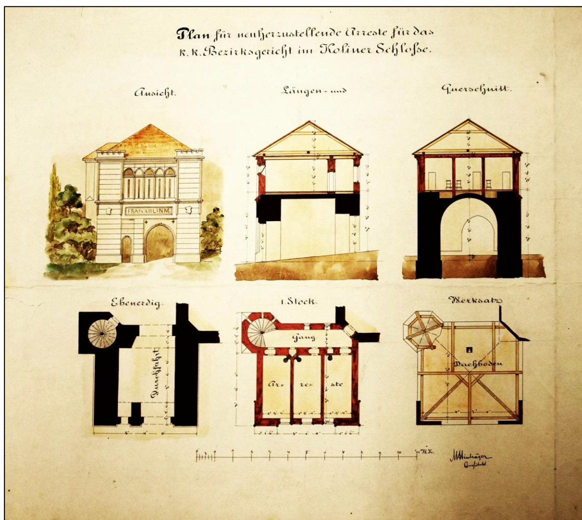
Plán na stavbu věznice okresního soudu v Kolíně, 60. l. 19. st. (foto: SOkA Kolín, f. Archiv města Kolín)
